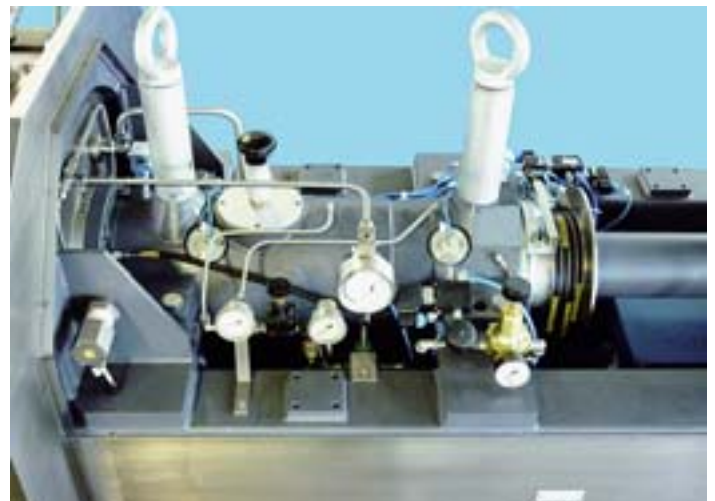
Das Innenleben einer Heinkel Stülpfilterzentrifuge beim Ankauf (links) und nach der Modernisierung und dem Austausch aller Verschleißteile
